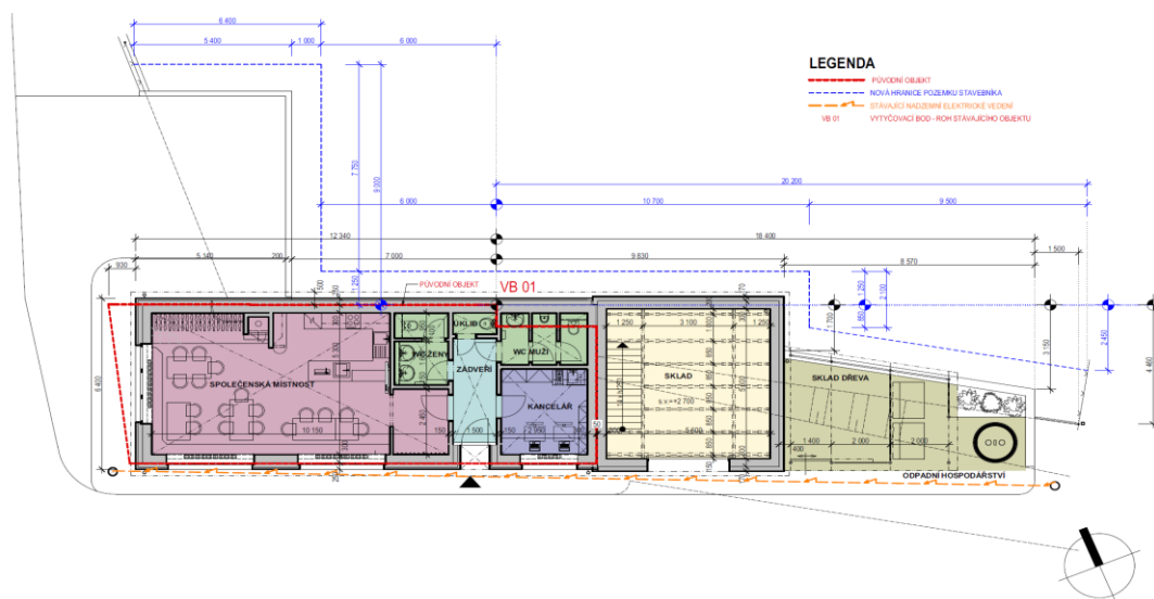
Půdorys nového stavu včetně přehledného zobrazení vnitřní dispozice
